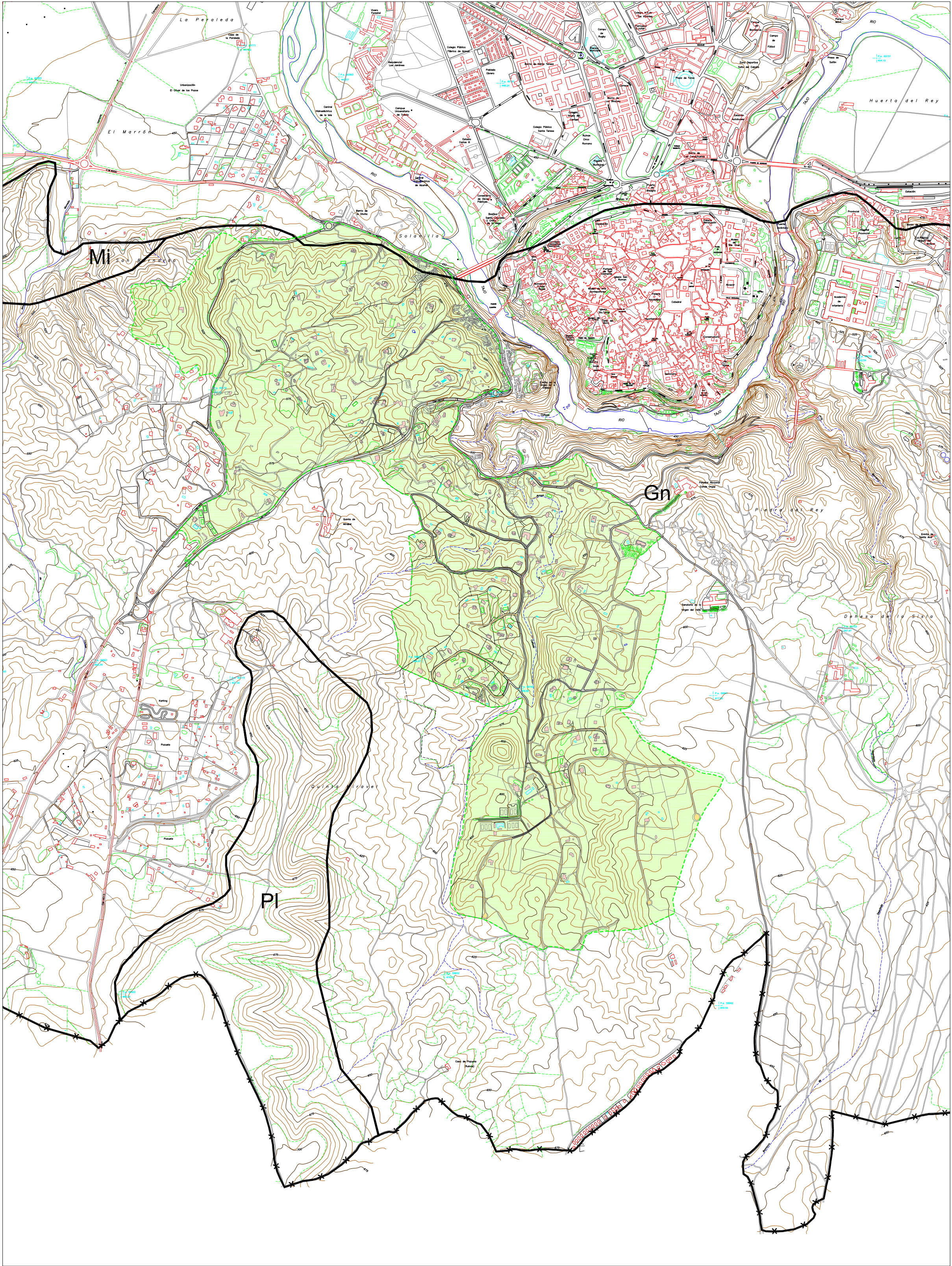
ESQUEMA LITOLÓGICO
